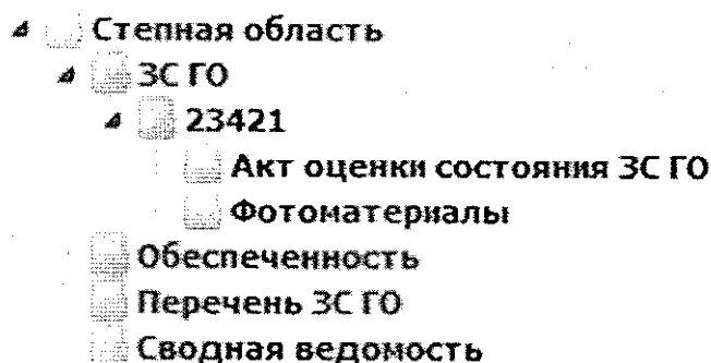
Рисунок 1 – Структура папок
